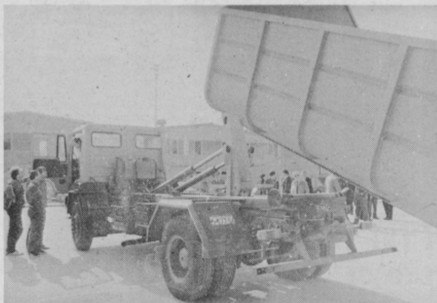
Emov kotalni prekucnik je nastal v sodelovanju s TAM Maribor.
