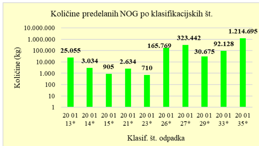
Slika 5: Količine predelanih nevarnih odpadkov iz gospodinjstev po klasifikacijskih št. odpadkov v kg.
