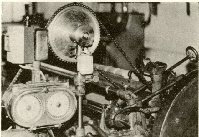
Slika prikazuje del škrobilnega stroja, na katerega bo vgrajena elektronska naprava za merjenje metraže blaga. Naprava bo tako izpopolnjena, da bo oddajala opozorilne signale ob nastavljeni količini metrov, nar kar bo delavec pri stroju tkanino odrezal.
