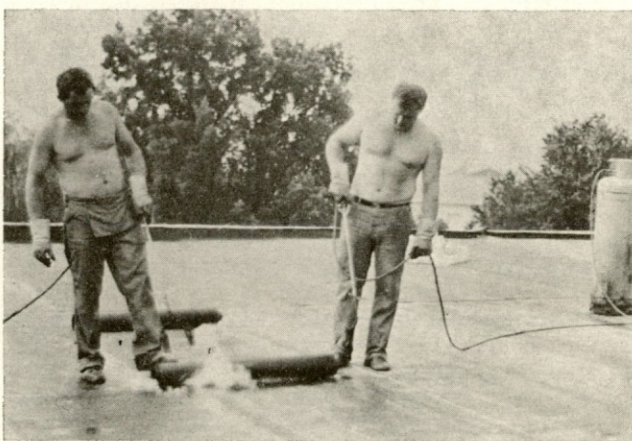
Zunanji izvajalci pri izvajanju hidroizolacije na strehi predilnice. Pri »nizki« temperaturi (okoli + 31° C) se delavca ogrevata s plinskim gorilcem.
