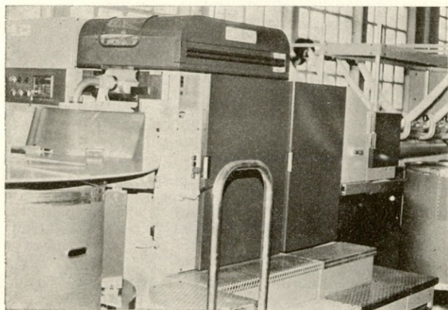
Med kolektivnim dopustom so v predilnici montirali nove Cognetex raztezalke.
