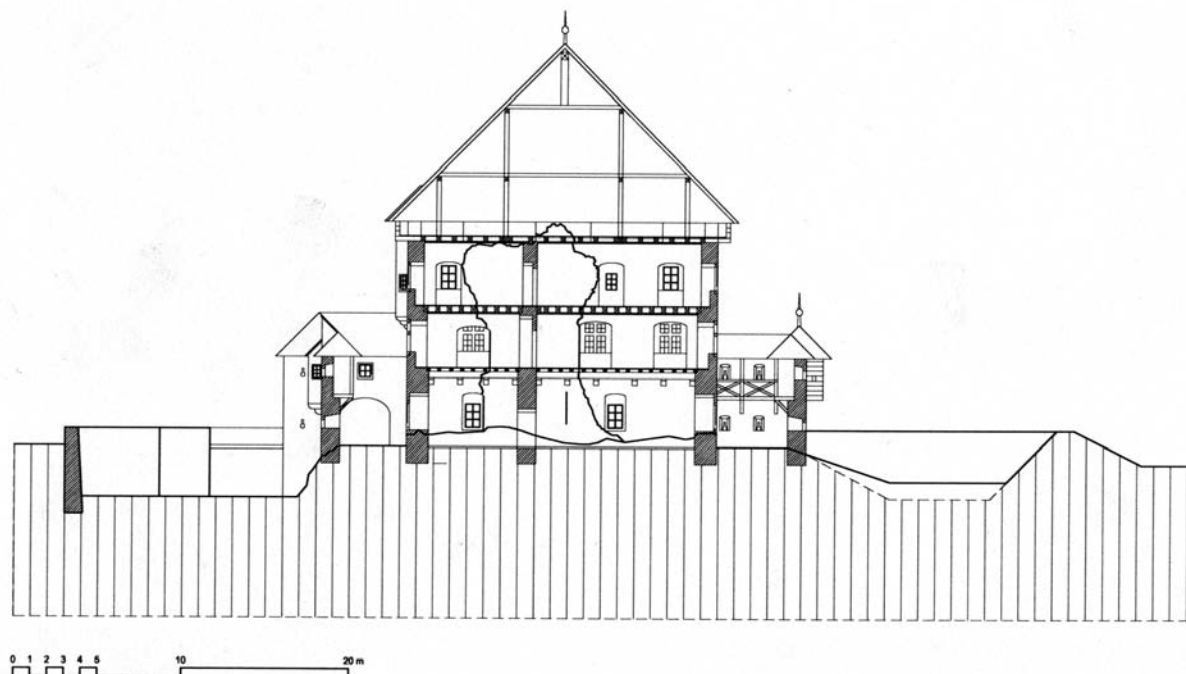
Prerez gradu Breg proti severovzhodu skozi glavno grajsko poslopje. Poskus rekonstrukcije (Igor Sapač. 2018).
