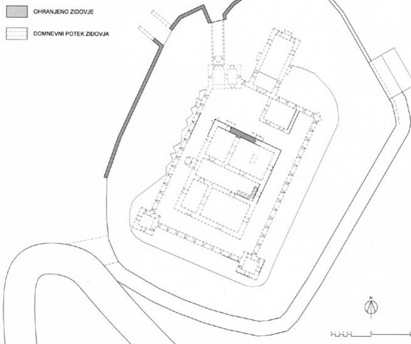
Tloris pritličja gradu Breg. Poskus rekonstrukcije z označenim ohranjenim zidovjem (Igor Sapač, 2018).
