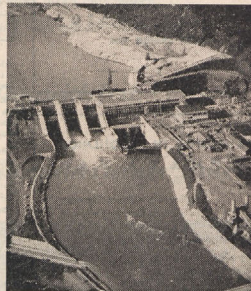
Draukraftwerk Feistritz i. R. 80.000 kW installierte Leistung, 375 Mill. kWh Jahresarbeitsvermögen, geht 1968 in Betrieb.
