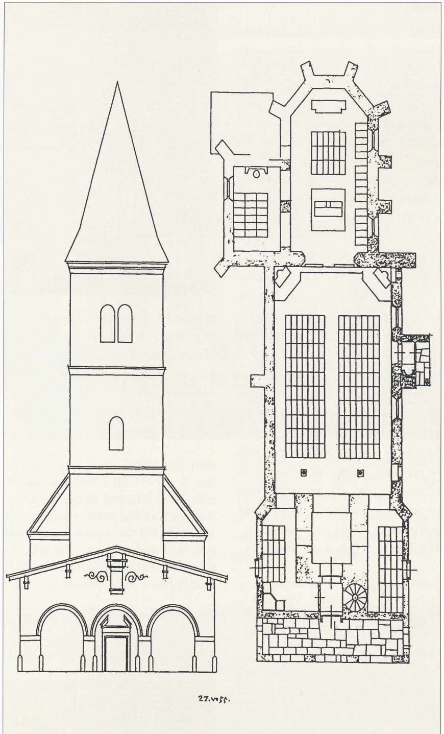
Tretji načrt, 27. julij 1955. Tloris cerkve in maketa pogledov z zahodne strani.
