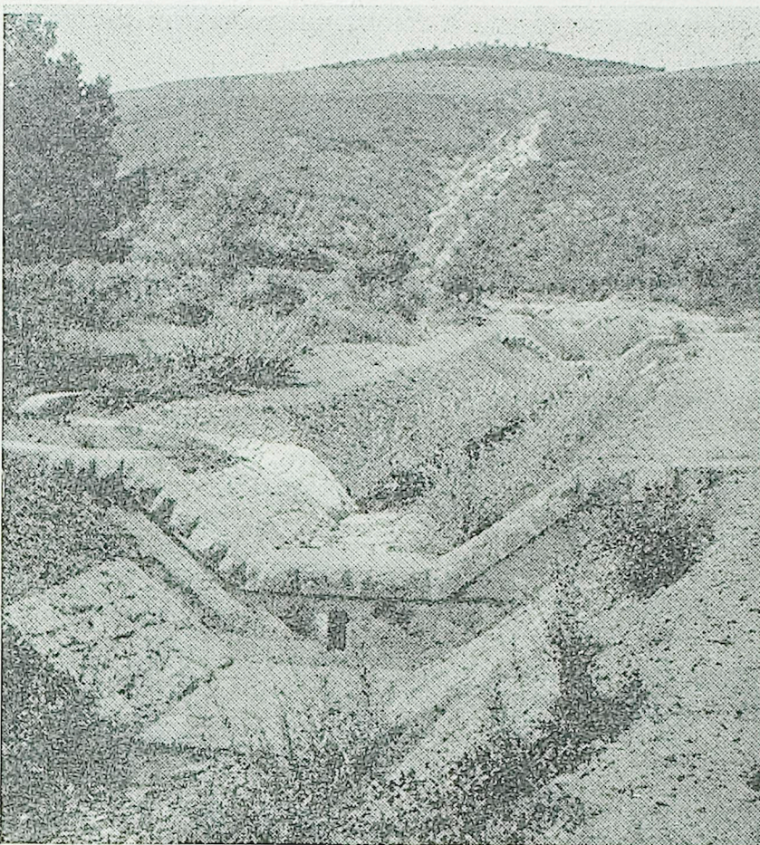
Sodobna ureditev in zavarovanje pogozdovanih površin pred divljanjem voda: urejena struga po naplavišču Trnovšice pri Ospu na Koprskem je zavarovana s pragovi in vrhovimi popletli brežin, ki utrjujejo zemljo, da je ne morejo odnesti hudourniški nalivi
