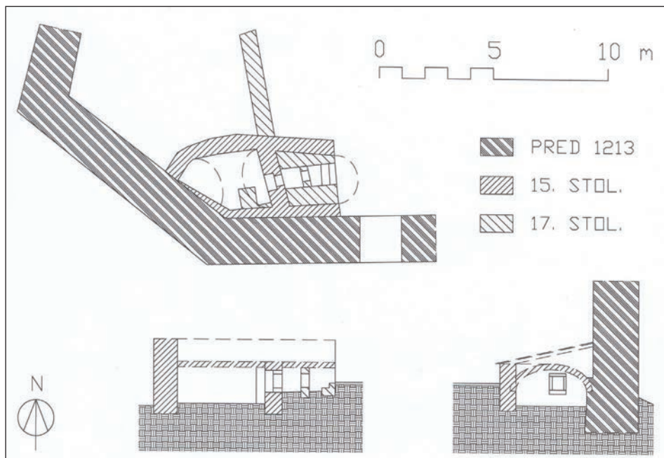
Sl. 27: Tloris, vzdolžni in prečni prerez izkopane srednjeveške ječe na notranjem grajskem dvorišču z označenimi stavbnorazvojnimi fazami in poskusom rekonstrukcije nekdanje strešne konstrukcije (po dokumentaciji iz ZVKDS OE Nova Gorica dopolnil in izrisal Igor Sapač).
