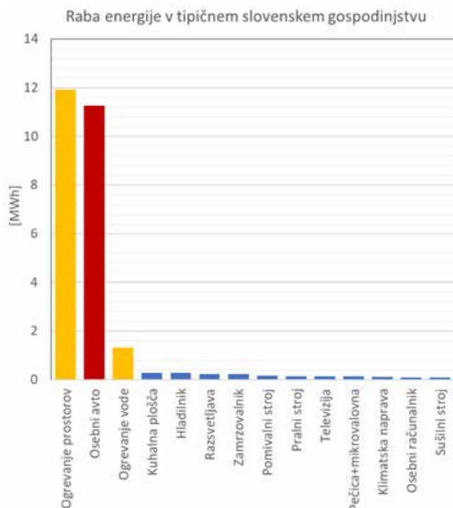
Slika 1: Ocenjena letna raba energije v tipičnem slovenskem gospodinjstvu: rumena-poraba zemeljskega
