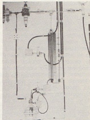
Merilna priprava za merjenje količine puščanja zaprtih posod z volumetrično metodo po GOS 359002 omogoča zelo precizna merjenja
