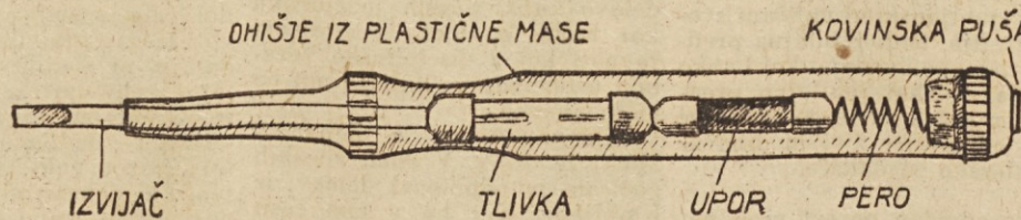
Indikator električnega toka v prerezu
