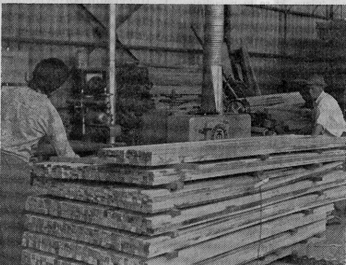
Sirinski narez pokončnikov in prečnikov ter skeleta za vhodna in garažna vrata na večlistni krožni žagi Torwegge v TO Mojstrana
