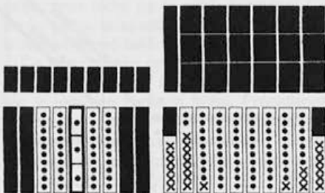
Shematičen prikaz namestitve trotovskega sata v AŽ panju z uporabo zaklade. V panju ni matične rešetke, zato ima matica dostop do vseh satov, ne more pa zalegati širokih mediščnih satov.
