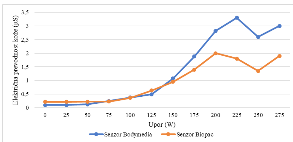
Slika 13: Povprečna električna prevodnost kože, merjena z merilnikom BodyMedia in Biopac
