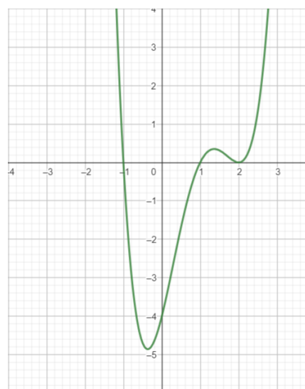
Graf polinoma 1
