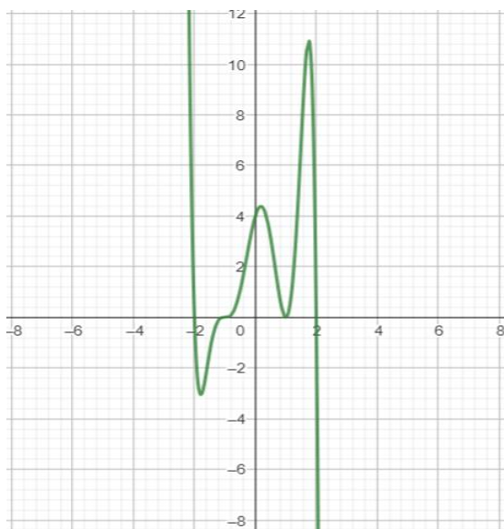
Graf polinoma 2
