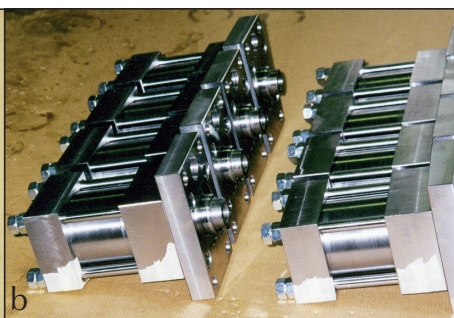
Hidravlični valji: a – s prirobnico, b – posebne izvedbe za visoke temperature
