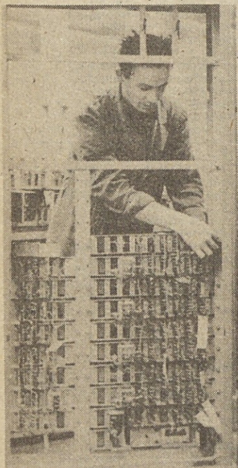
Telefonska centrala 4/30 je bila tudi sad prizadevanja ing. Šinkovca za razvoj Iskrine telefonije.
