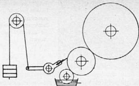
Shematičen prikaz strgala (rakla)
