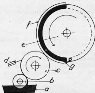
Šematičen prikaz tiskanja bakrotiska
