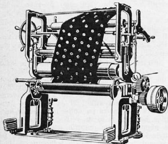
Stroj za tiskanje na katun
