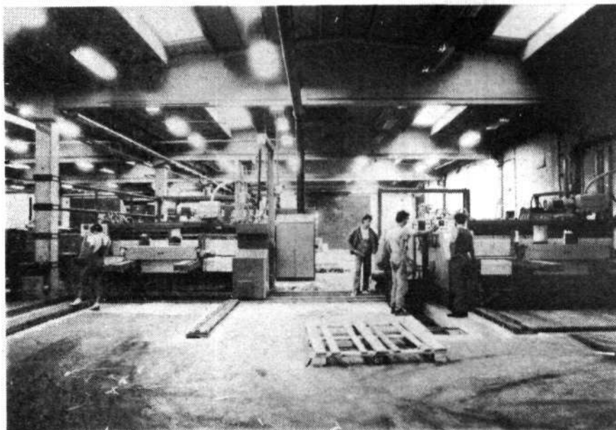
Oba dela novega stroja — izdelovalec škatel in rotacijska stanca — sta povezana s tiri, po katerih je omogočena izmenjava posameznih segmentov stroja. (Foto: Črt Čargo)
