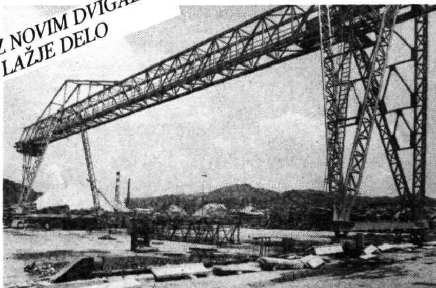
Novo portalno dvigalo, ki je panično po tračnicah, bo pokrivalo prostor v dolžini 330 in v širini 50 metrov. (Foto: Črt Čargo)
