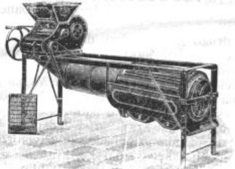
Pod. 26. Univerzalni čistilni in sortirni stroj za žito.
