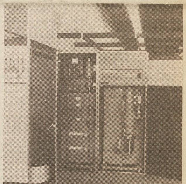
Prvi desetkilovatni televizijski UHF oddajnik. IMP je še vedno edini jugoslovanski proizvajalec TV oddajnikov.
