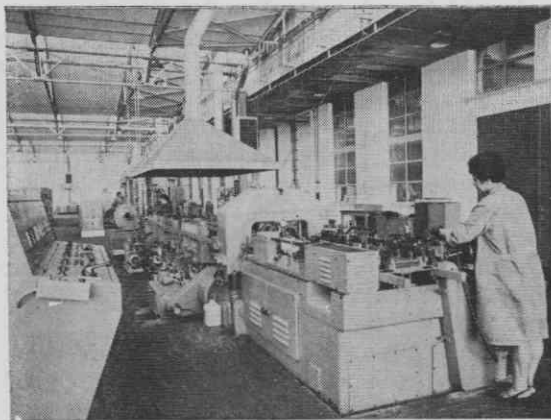
Nova linija za izdelovanje konzervnih škatel z zmogljivostjo do 9000 kosov na uro, postavljena v obratu Zalog, specializiranem za proizvodnjo konzerv
