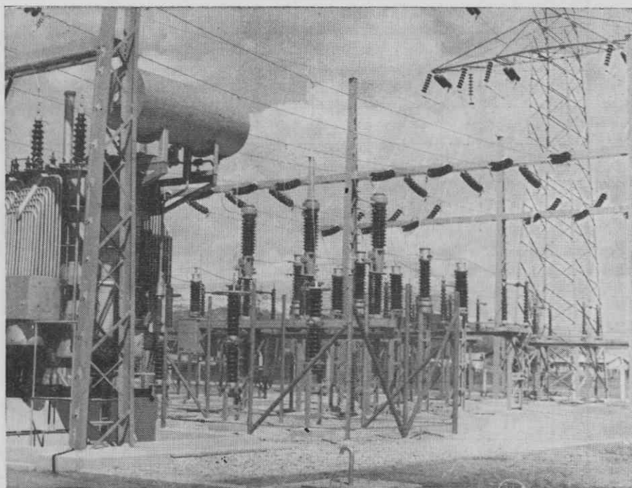
RTP Ljubljana-Siška 110 kV stikalo
