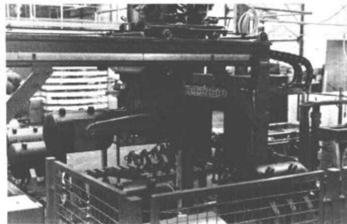
Večji ekonomski prihranki v proizvodnji, bistveno višja kakovost grelnikov vode, izboljšanje delovnih pogojev in povsem odpravljeno težko fizično delo so rezultati avtomatizacije (na sliki) montažne linije v proizvodnji električnih grelnikov vode v Gorenju Tiki, za katero so strokovnjaki Gorenja Procesna oprema prejeli Kidričeve nagrade.
