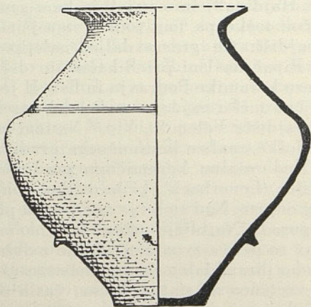
Velika shrambena posoda, inv. štev. 28377. Vel. 1:12
