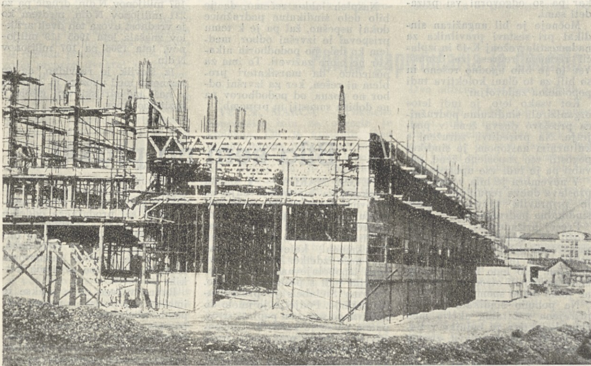
Zgradba za premazni stroj dobiva obliko. Takole je izgledala 15. II. 1967 — pogled z južne strani. (Foto: Ocvirk)
