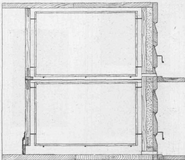
Pod. 7. Podolžni prerez.
