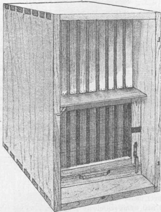
Pod. 1. Zadaj odprti panj.
