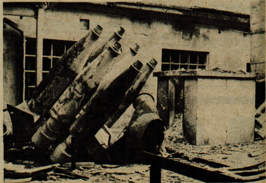
Šestceveni ciklon (na fotografiji) tvori srce prežračevalne naprave, ki jo sestavljata še sistem odvajalnih cevi ter betonski silos. Vžig drobcev v njej je povzročil prašno eksplozijo z znanimi posledicami — Foto: M. K.
