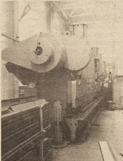
Ogromna stiskalnica za dvojno upogibanje lahko upogiba tudi do 12 m doleže kose.
