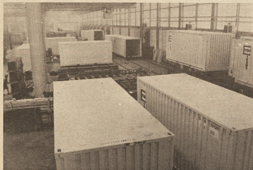
Panorama montažnega dela proizvodne dvorane.
