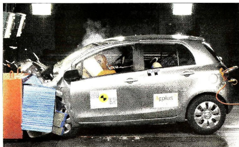
Toyota yaris ob preskusnem trčenju
