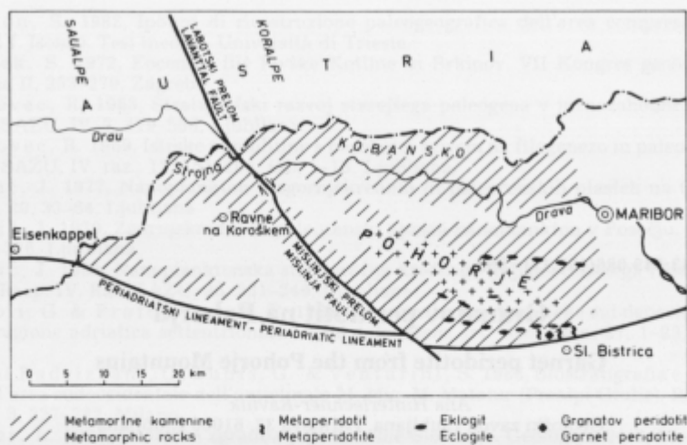
Sl. 1. Shematsko nakazana razširjenost metamorfnih kamenin Vzhodnih Alp v Sloveniji. Osrednji del Pohorja sestavlja tonaltni pluton (+). Nakazana so nahajališča metaperidotita, eklogita in granatovega peridotita
