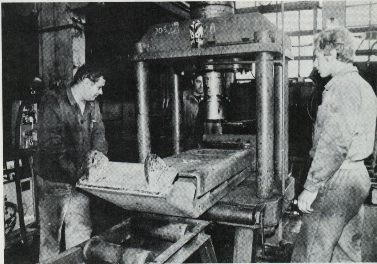
Nov tehnološki postopek izdelave podpora hemscheidt v TOZD ESO, katerega avtorji so Ivan Zupančič, Franc Pečečnik in Miha Letonje. Z rekonstruiranjem 150-tonske stiskalnice in izdelavo funkcionalnega orodja (Na sliki!) so od prej toplega krivljenja pločevine prešli na hladno in s tem produktivnost pri tem postopku povečali več kot 4-krat. Celotni ekonomski prihranek racionalizacije še niso ugotovili, zato nagrade avtorjem še niso določene.
