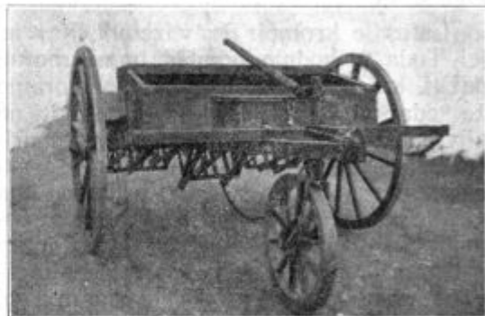
Slika 38. Sejalni stroj domačega izdelka (Jos. Peternelj, Selca nad Škofjo Loko 67); pogled od spredaj.
