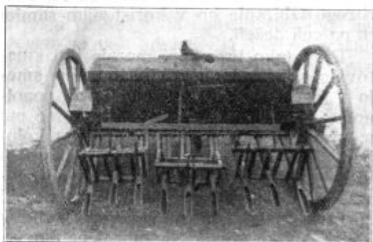
Slika 39. Peterneljev sejalni stroj; pogled od zadaj.
