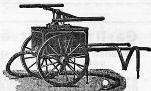
Dvokolna brizgalnica, podvojevo brizgajoča 180 — 200 2/min.
