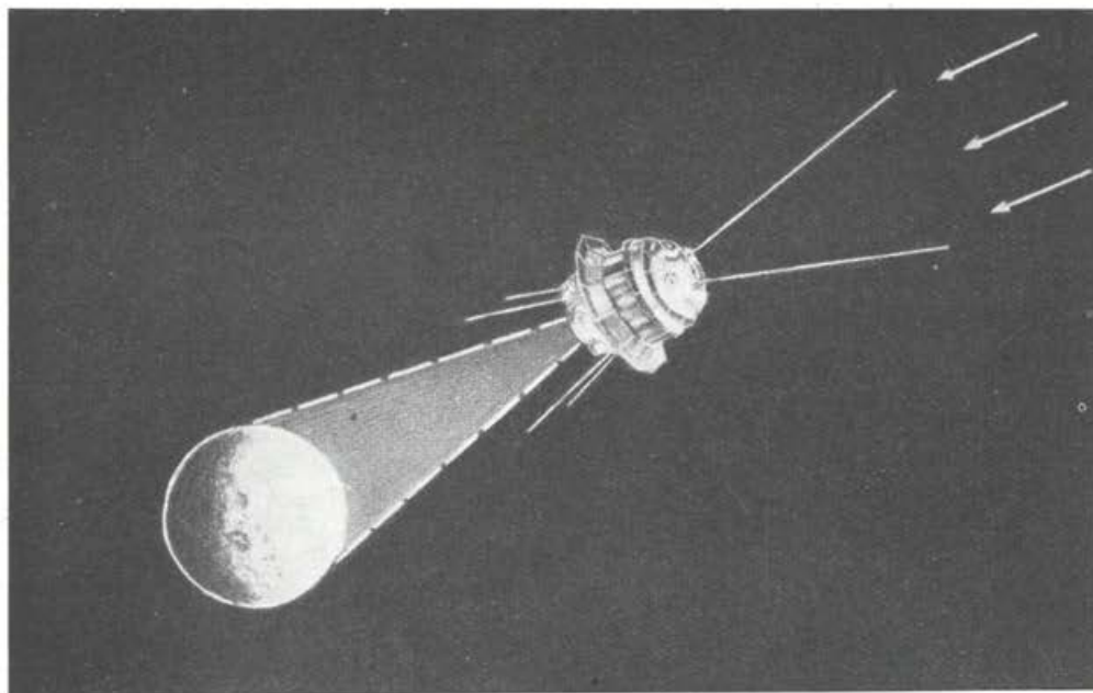
Položaj Lunika III v medplanetnem prostoru pri fotografiranju zadnje plati Lune. Puščice na desni kažejo smer sončnih žarkov.
