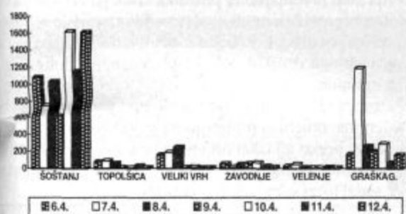
MAKSIMALNE POLURNE KONCENTRACIJE SO 2 od 6.aprila do 12.aprila 1998
