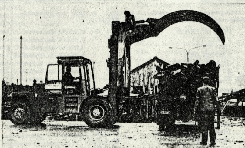
Močan viličar naloži tovor celega kamiona naenkrat. Posneto v Slovenj Gradcu.
