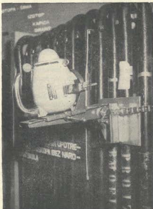
Naprava z radioaktivnim izotopom za preiskovanje kovinskih cevi pri cevovodih, parnih kotlih in podobno. (Izdelek podjetja »Energoinvest«, Sarajevo)
