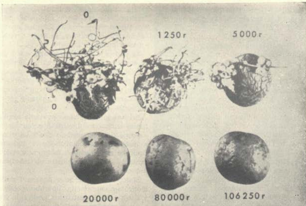
Radioaktivne izotope lahko uporabljamo s pridom tudi pri konserviranju raznih živil. Na sliki je razvidna kaljivost krompirja po obsevanju z različnimi dozami radioaktivnih žarkov. S primernimi dozami lahko kaljivost popolnoma preprečimo
