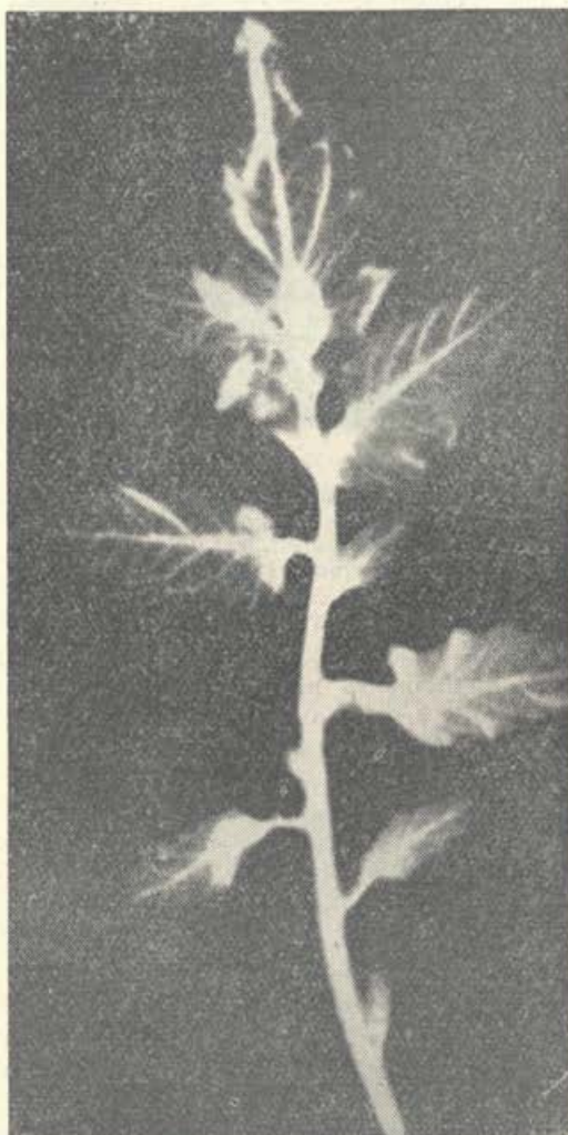
Uporaba radioaktivnih izotopov v agronomiji. Na sliki vidimo razporeditev radioaktivnega fosfora v listih in stebelu rastline. Z radioaktivnim fosforom je bilo zaznamovano umetno gnojilo, ki ga je črpala rastlina iz zemlje. Tako lahko z radioaktivnimi izotopi preiskujemo prehrano in rast rastlin
