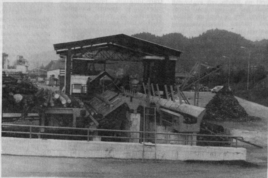
Na prvi komandni mizi daje delavec komande za delovanje prečnega transporterja, vzdolžnega transporterja, stroja za lupljenje in transport oblovine skozi merilne naprave
