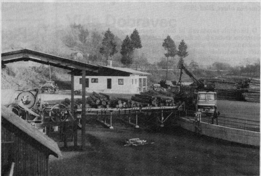
Nakladanje oblovine na sprejemni transporter za razdelitev te in dodajanje na vzdolžni transporter, ki vodi do stroja za lupljenje in k merilnim napravam. V ozadju novi prostori za potrebe delavcev s priročno delavnico in lopa za viličarje
