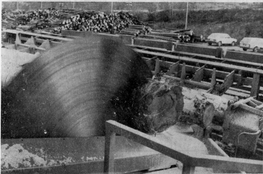
Sistem treh krožnih žag omogoča, da je hlodovina očeljena in razžagana na pravilne dolžine
