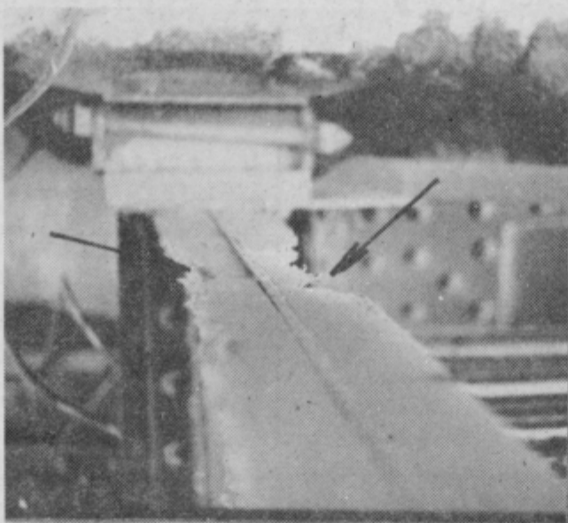
Popolnoma uničen glavni nosilec mostu
