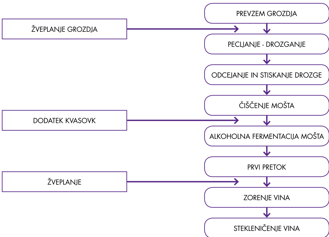
Slika 1: Shema pridelave belega vina iz belega grozdja Vir: lastni 2020 po Bavčar 2020, 15–143
