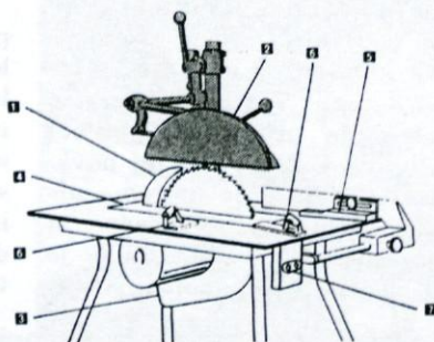
1. razporni klin; 2. zaščitna kapa; 3. odsevalno ustje za žagovino; 4. vložek; 5. vodilo; 6. pripomočki za potiskanje; 7. stikalo
