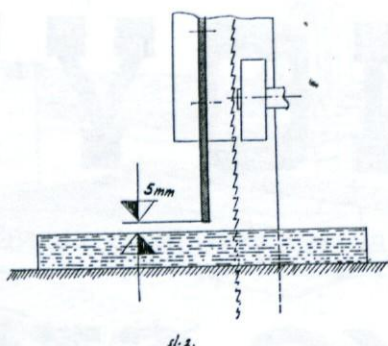
Gibljiva zaščita tračne žage
