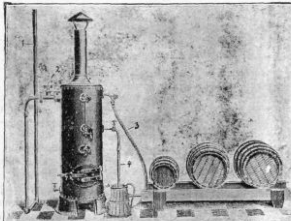
Podoba 14. Kotel za izparjenje sodov pri delu. Ta kotel daje ne samo sopar, ampak tudi vrel krop.
