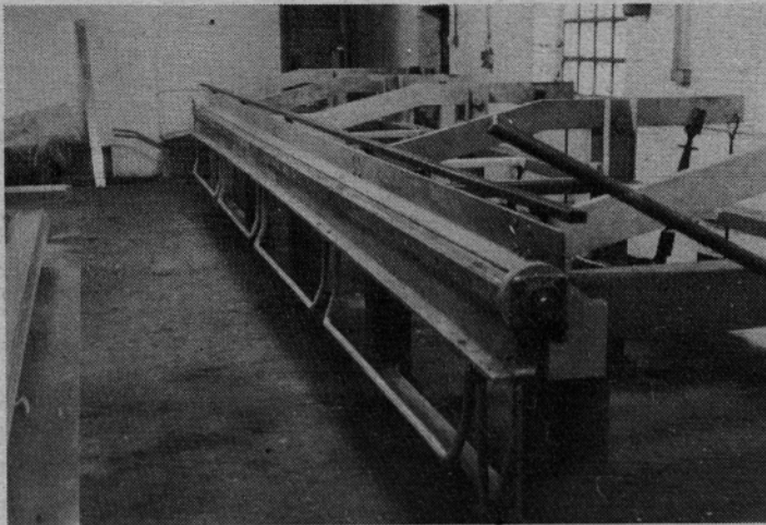
Kovinski delavci Komunalnega podjetja so si pomagali, ko so sami naredili stroj za krivljenje pločevine večjih razsežnosti. Tako so prihranili drago prevažanje pločevine v Celje, sedaj lahko ta dela opravijo kar doma.
