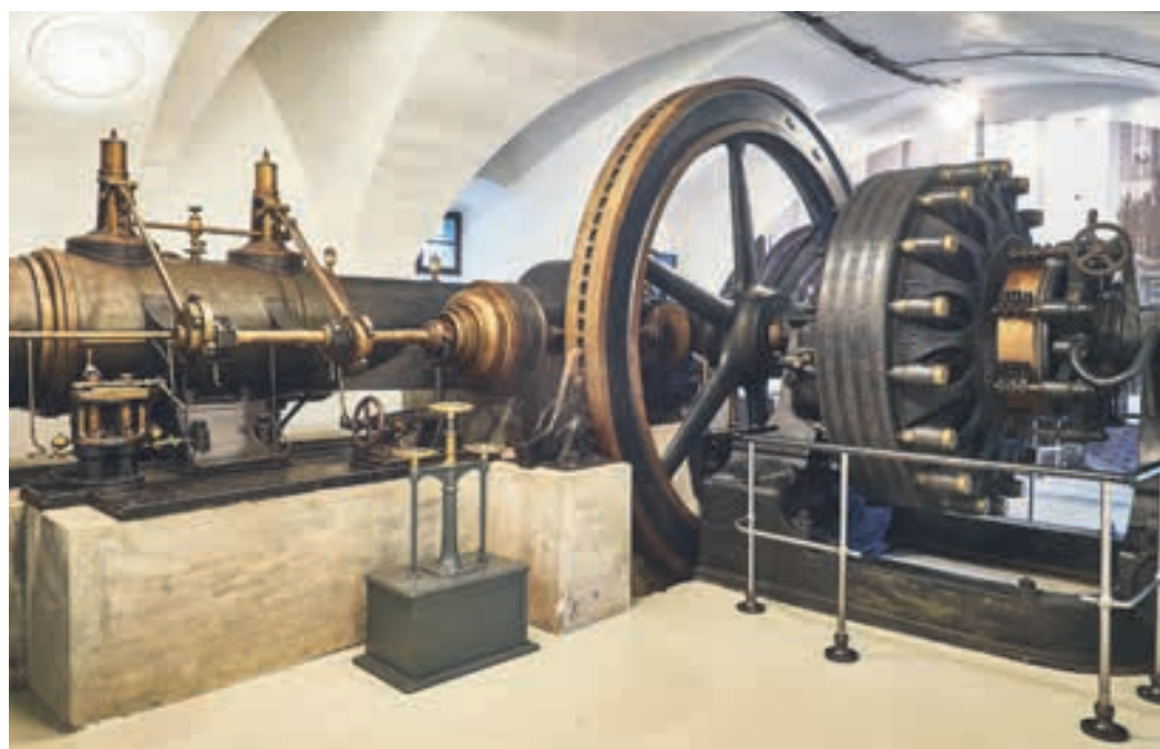
Parni stroj in generator iz Mestne elektrarne Ljubljana. Parni stroj je izdelala Prva brnska tovarna strojev, enosmerni generator s 120 kW moči pa je delo dunajske tovarne Siemens-Halske. V Ljubljani je prva električna luč zasvetila leta 1898 (foto: Dragan Arrigler).
