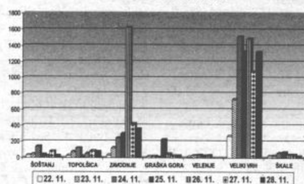
MAKSIMALNE POLURNE KONCENTRACIJE SO 2 od 22. novembra do 28. novembra 1999
