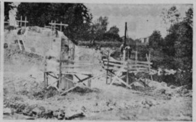
Ljubljanski Gradis, TOZD nizke gradnje Maribor, gradi most čez Savinjo v Latkovi vasi. Na posnetku vidimo dva stebra, ki bosta nosila konstrukcijo novega železobetonskega mostu. Zadnje močne deževje je povzročilo graditeljem nekaj škode. Navzlec temu upajo, da bodo dela pravočasno končali. TONE TAVCAR
