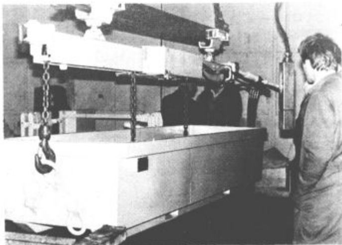
Eden od petih prototipnih izdelkov, ki jih bodo najprej preizkusili v Rudniku lignita Velenje je tudi novi voziček kontejnerske izvedbe. (fotografija B. M.)
