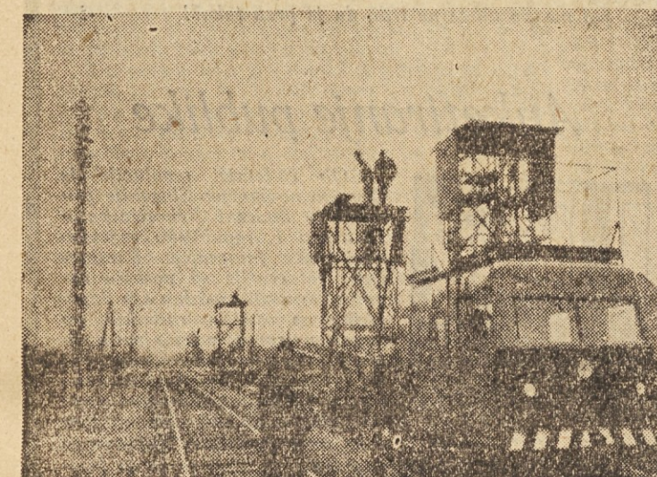
Te dni montirajo napeljavo za popolno elektifikacijo proge Postojna-Ljubljana že tik pred Ljubljano. Zica je napeljana že do Dolgega mostu, nosilce pa montirajo v Rožni dolini (slika). Zaradi tehničnih del vozijo vlaki na tem odseku le po enem tiru. Vse to obeta, da se z gotovostjo bližamo dnevu, ko bodo tudi v Ljubljani zatulile sirene električnih lokomotiv in ko bodo po vseh naših važnejših progah zamenjale žice črni dim starih lokomotiv, čeprav se niso končala prerekanja o tem, kakšen sistem napajanja naj velja na naših progah.
