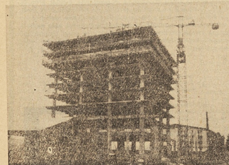
V Zalcu so septembra meseca začeli graditi novo najsodobnejše skladišče hmelja v Evropi. V njem bodo dosuševali, konservirali, pakirali ter odpošiljali hmelj. Nova gradnja, ki bo predvidoma gotova do konca 1962. leta, bo visoka čez 50 m, vsi delovni poslopki v njej pa bodo avtomatizirani. Zmogljivost novega skladišča bo 650 ton hmelja za predelavo ter 200 ton že prepranega. Po novem tehnološkem postopku, ki je edinstven na svetu in izključno izum naših tehnologov, bodo osemkrat povečali storilnost zveplanja, izboljšali kvaliteto hmelja, obenem pa prihranili samo na zveplu nad 90 %
