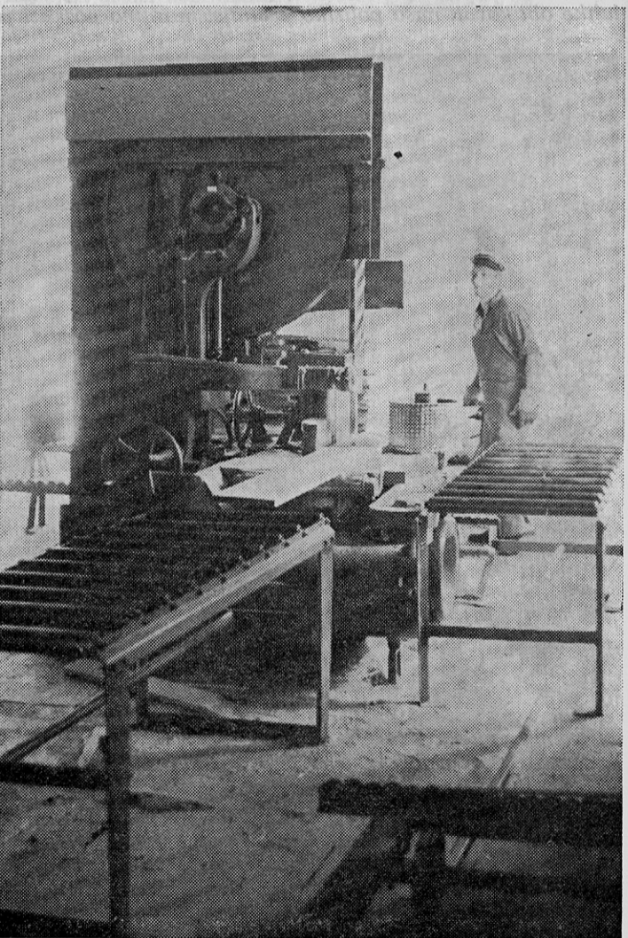
Tračna žaga v TOZD Rečica
