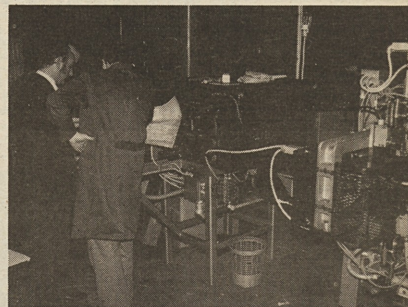
TOZD ELEKTROMOTORJI ŽELEZNIKI: Te dni montirajo nov avtomatski stroj – kombiniran za vlaganje utorne izolacije in navijanje statorjev. Stroj je uvožen iz ZDA – firma GLOBE, povečal bo kvaliteto dela, omogočil hitrejši tempo proizvodnje in bo zamenjal najmanj tri delavke.
